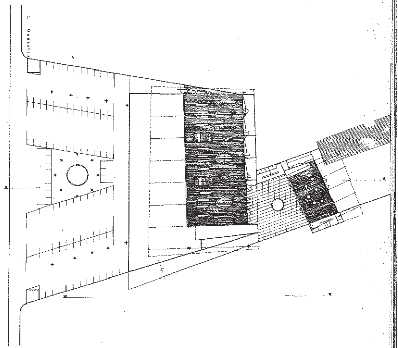
planta -3m / -3m floor plan
