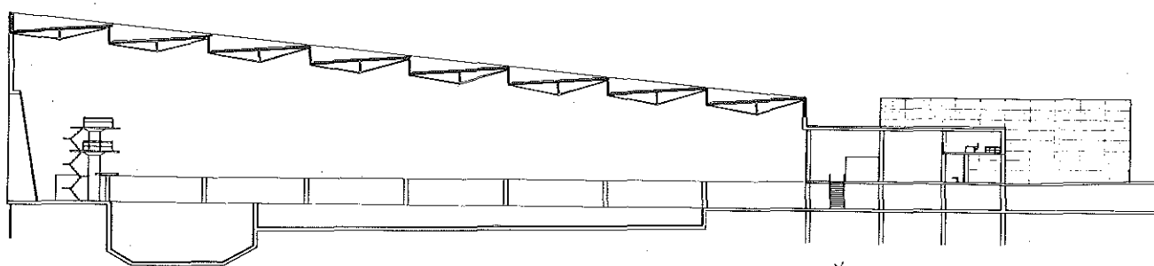
sección longitudinal longitudinal section
