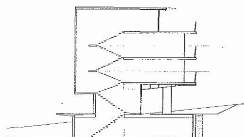
sección del edificio de viviendas. section of the housing building
