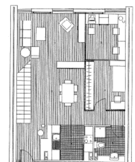
vivienda tipo e type dwelling e
