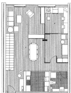
vivienda tipo b type dwelling b
