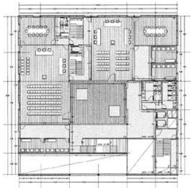
planta primera first floor
