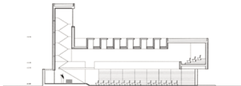
sección d section d
