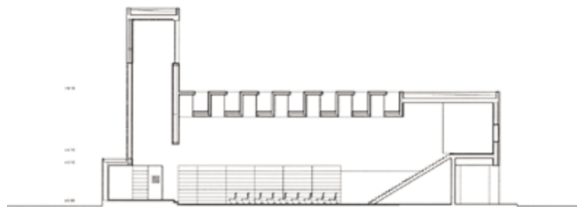
sección c section c
