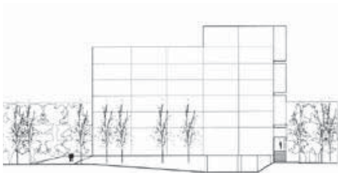
alzado este east elevation
