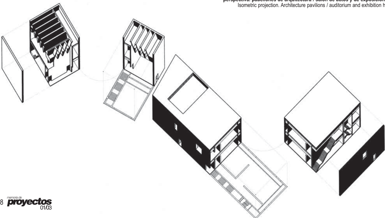
perspectiva. pabellones de arquitectura / salón de actos y de exposiciones Isometric projection. Architecture pavilions / auditorium and exhibition hall
