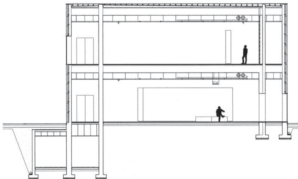
galería de exposiciones. sección transversal exhibition gallery. cross section
