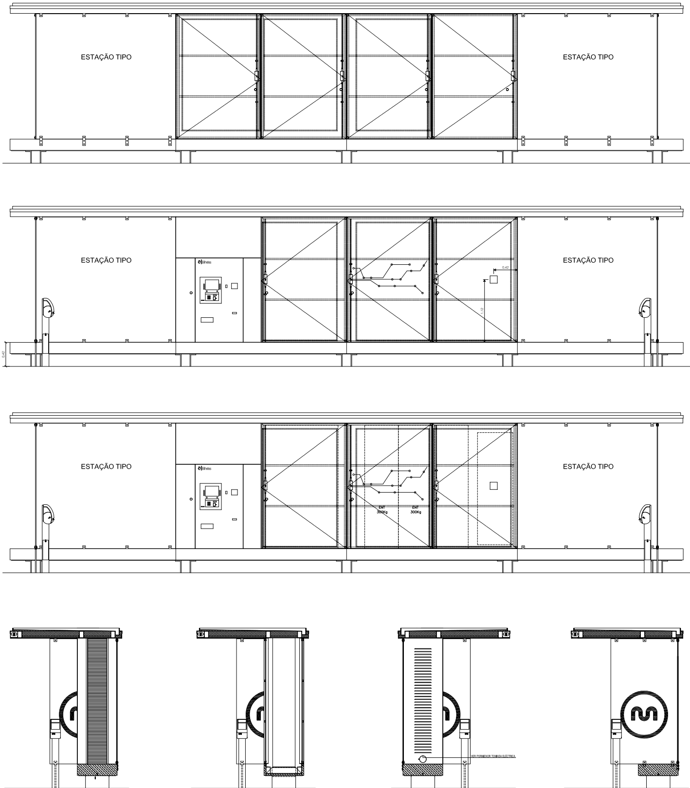
Plantas, alzados y secciones de marquesina urbana tipo
