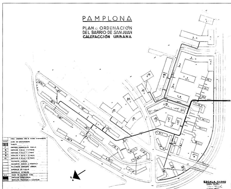
Plano de la instalación en el barrio del Tercer Ensanche ("Barrio de San Juan" en el plano)
