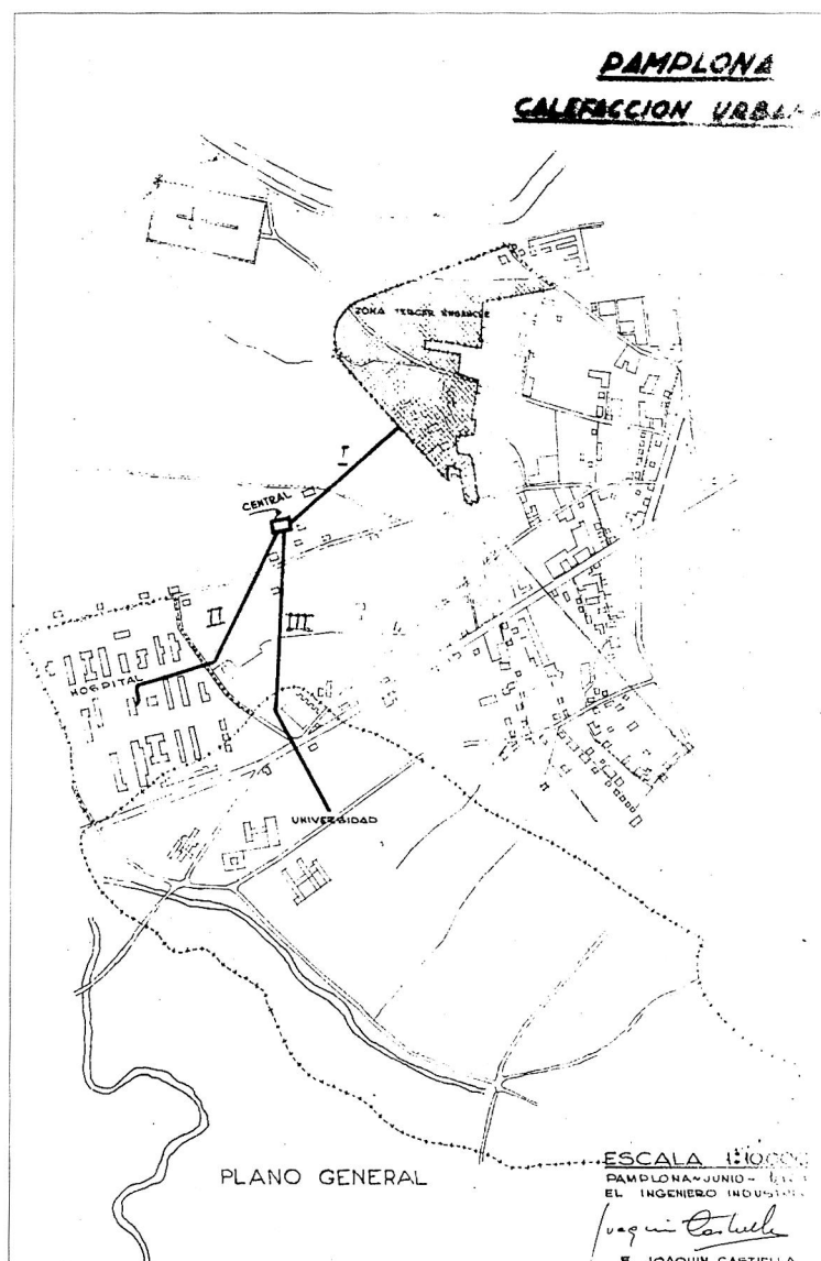
Plano general de la actuación prevista en el proyecto, con la ubicación de la central térmica en relación a los tres ámbitos de actuación
