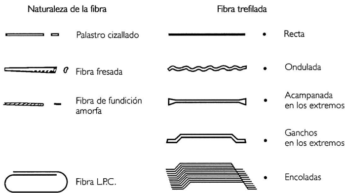
7. Diversas formas geométricas de las fibras metálicas
