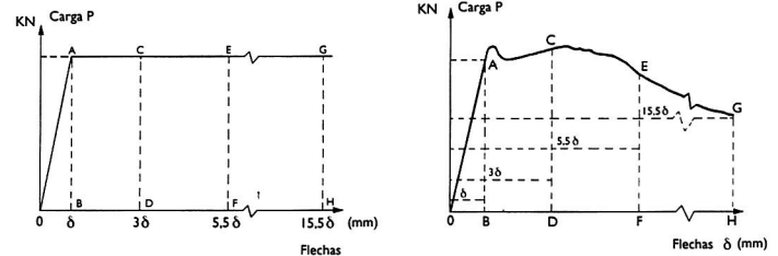
2. Diagrama carga-flecha para un material elasto-plástico
