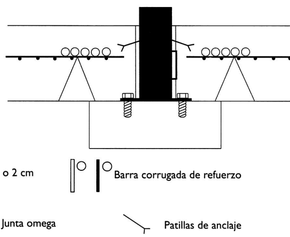
16. Detalle de refuerzo de pilar con cruce de omega
