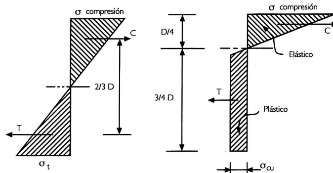
18. Diagrama rectangular de tensión de tracción según Edington
