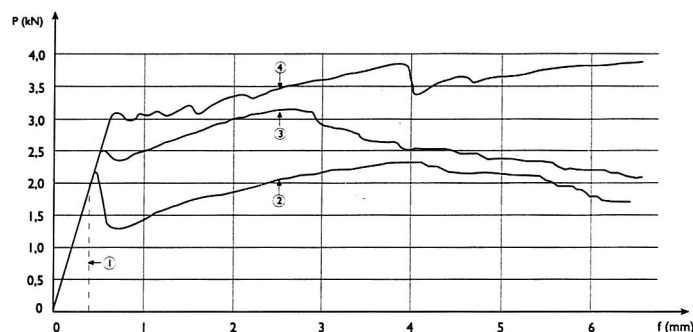
17. Curvas carga-flecha en esfuerzo de flexión
