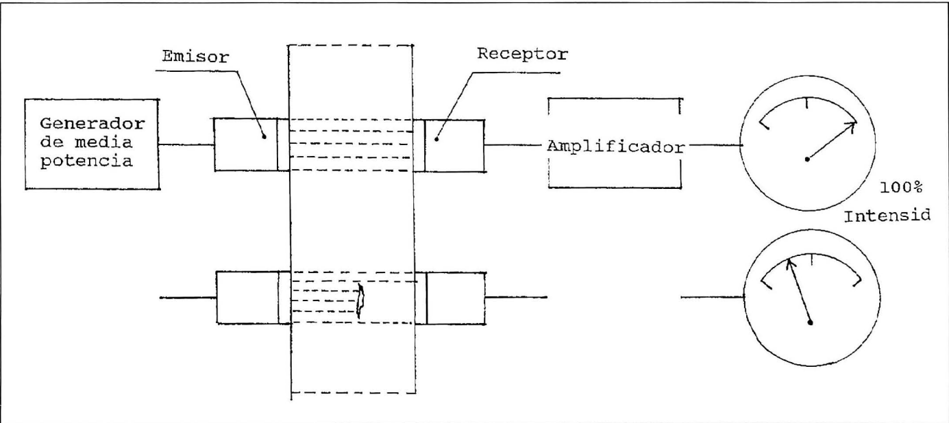
Figura 6 Método de inensidad con transmisión del sonido
