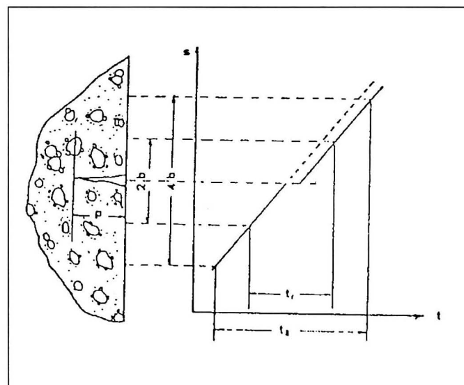
Figura 14 Medición de la profundidad de una grieta
