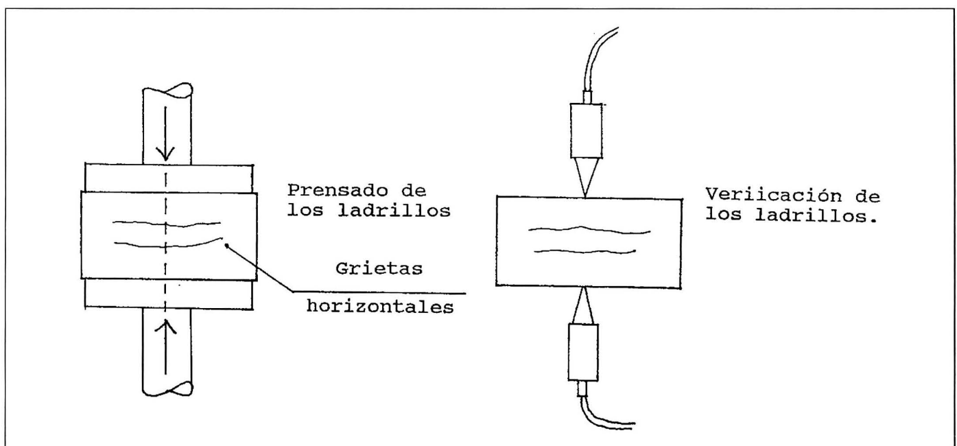
Figura 16 Formación de grietas en ladrillos refractarios
