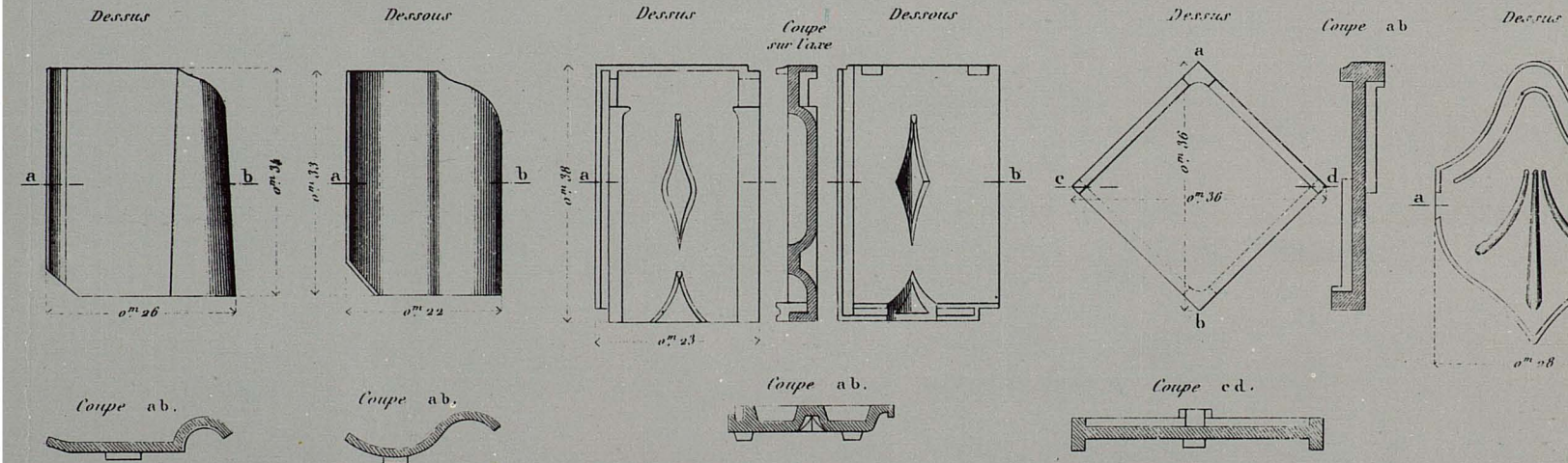
Fig. 6. Tuile Gérard. (poids 2 k 260.)
