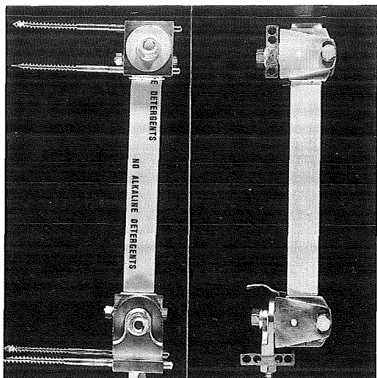
Fig. 9.—Aparato de Wagner modificado por Cañadell.
